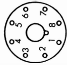
Mazda Octal (M08)
